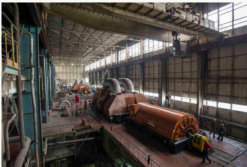
Une vue de l'intérieur de la centrale thermique Kosovo A.
